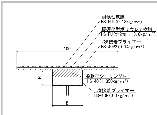
施工断面図
